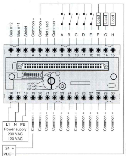
Type / Unit : 24 VDC ICSO 08 R1 Binary output module
