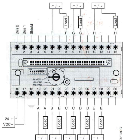
Type / Unit : 24 VDC ICSO 08 R1 Binary output module
