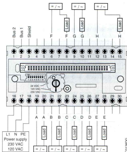
Type / Unit : 24 VDC ICSO 16 N1 Binary output module
